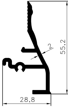
Pr.No: 8826 0,607 kg/m ÖZEL/PRIVATE
