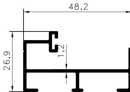
Pr.No: 9488 1,400 kg/m ÖZEL/PRIVATE
