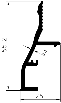
Pr.No: 8825 0,504 kg/m ÖZEL/PRIVATE
