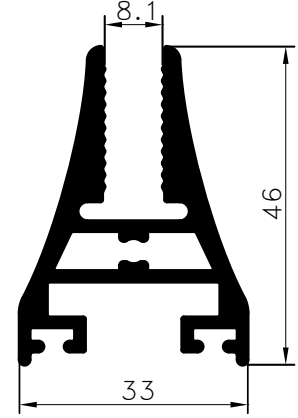
Pr.No: 9308 1,104 kg/m ÖZEL/PRIVATE
