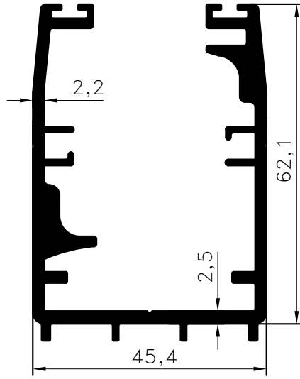
Pr.No: 9114 1,623 kg/m ÖZEL/PRIVATE
